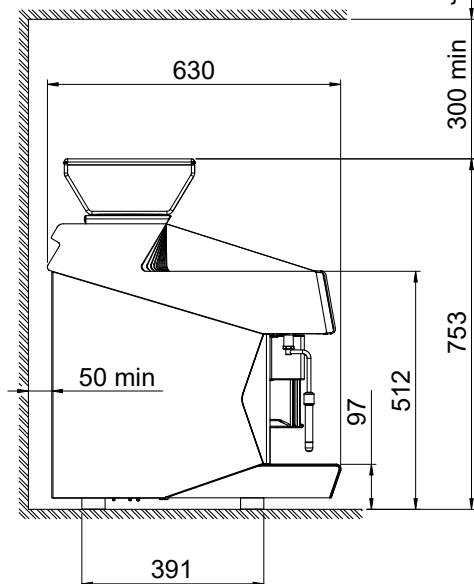
Zij aanzicht
